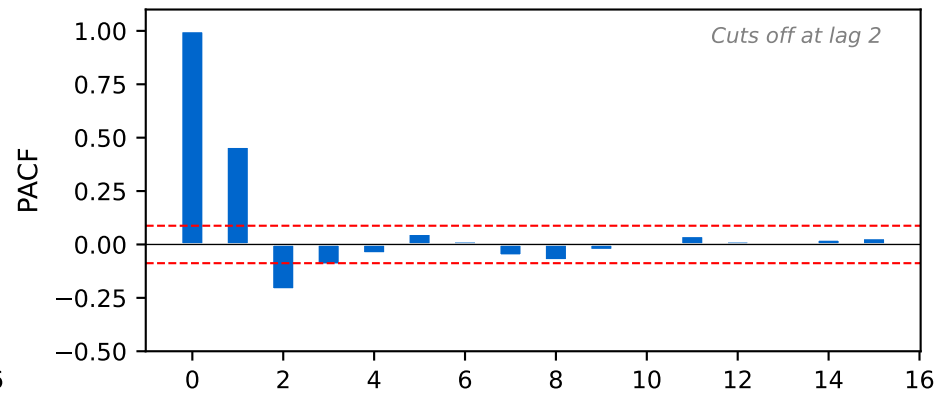
PACF
