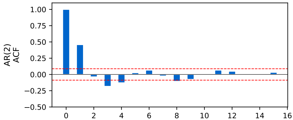
ACF
