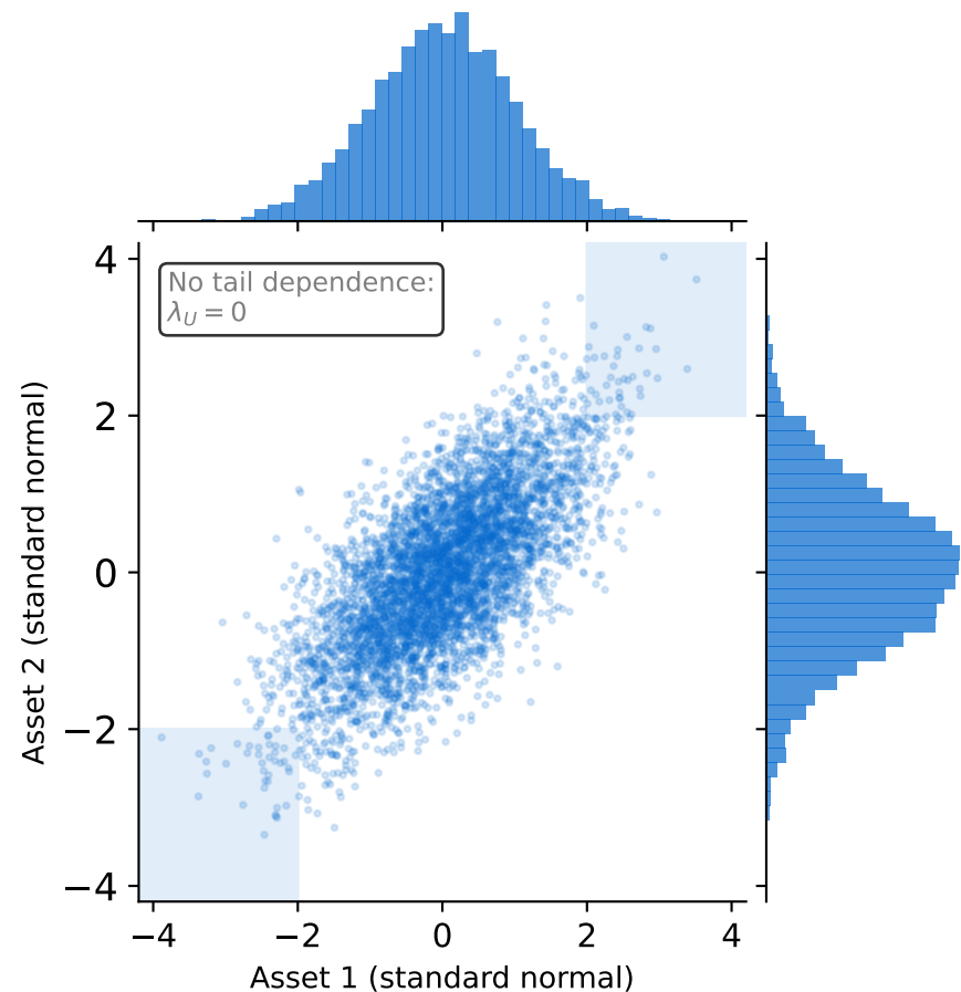
Gaussian Copula ( \rho = 0.7 )
