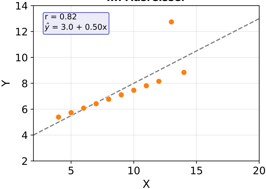
III: Ausreisser
