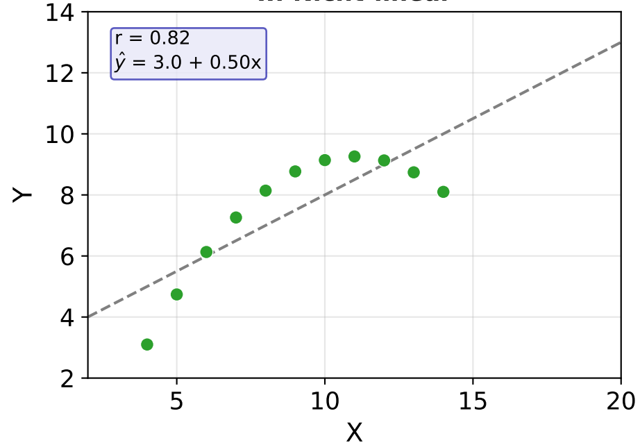
II: Nicht-linear
