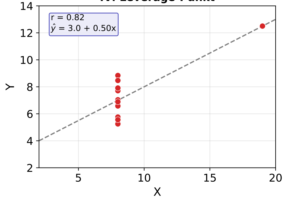
IV: Leverage-Punkt
