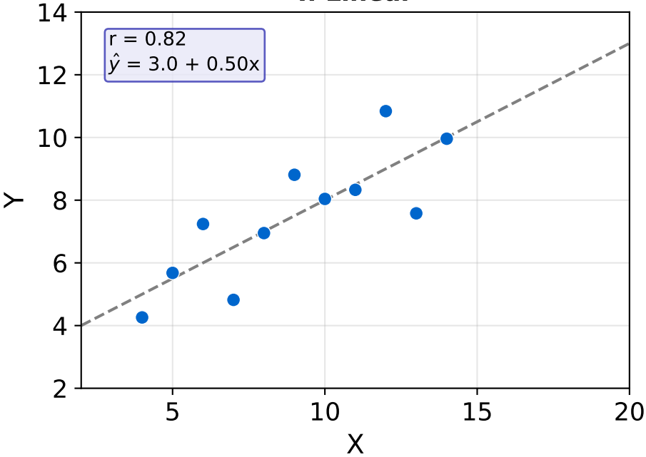
I: Linear
