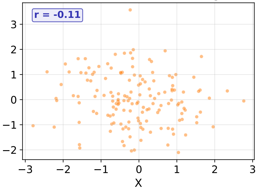
r = 0.0 (kein Zusammenhang)
