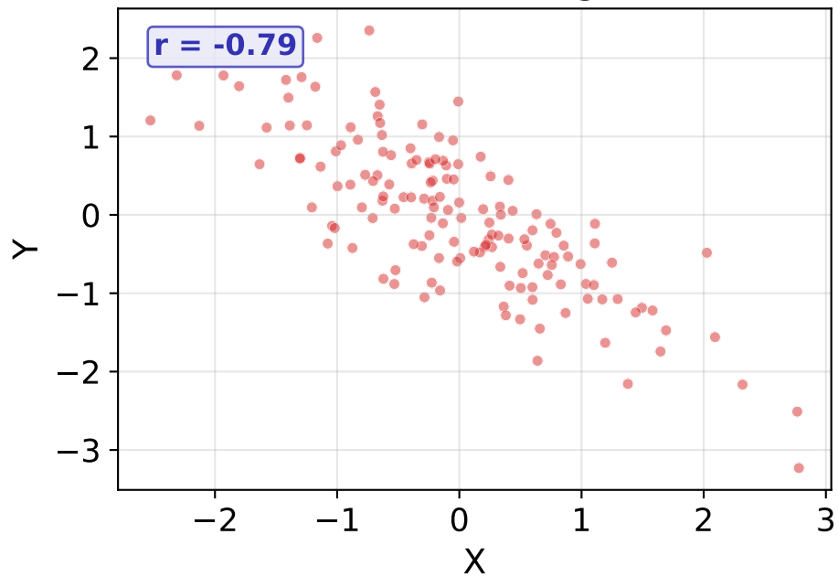
r = -0.8 (stark negativ)
