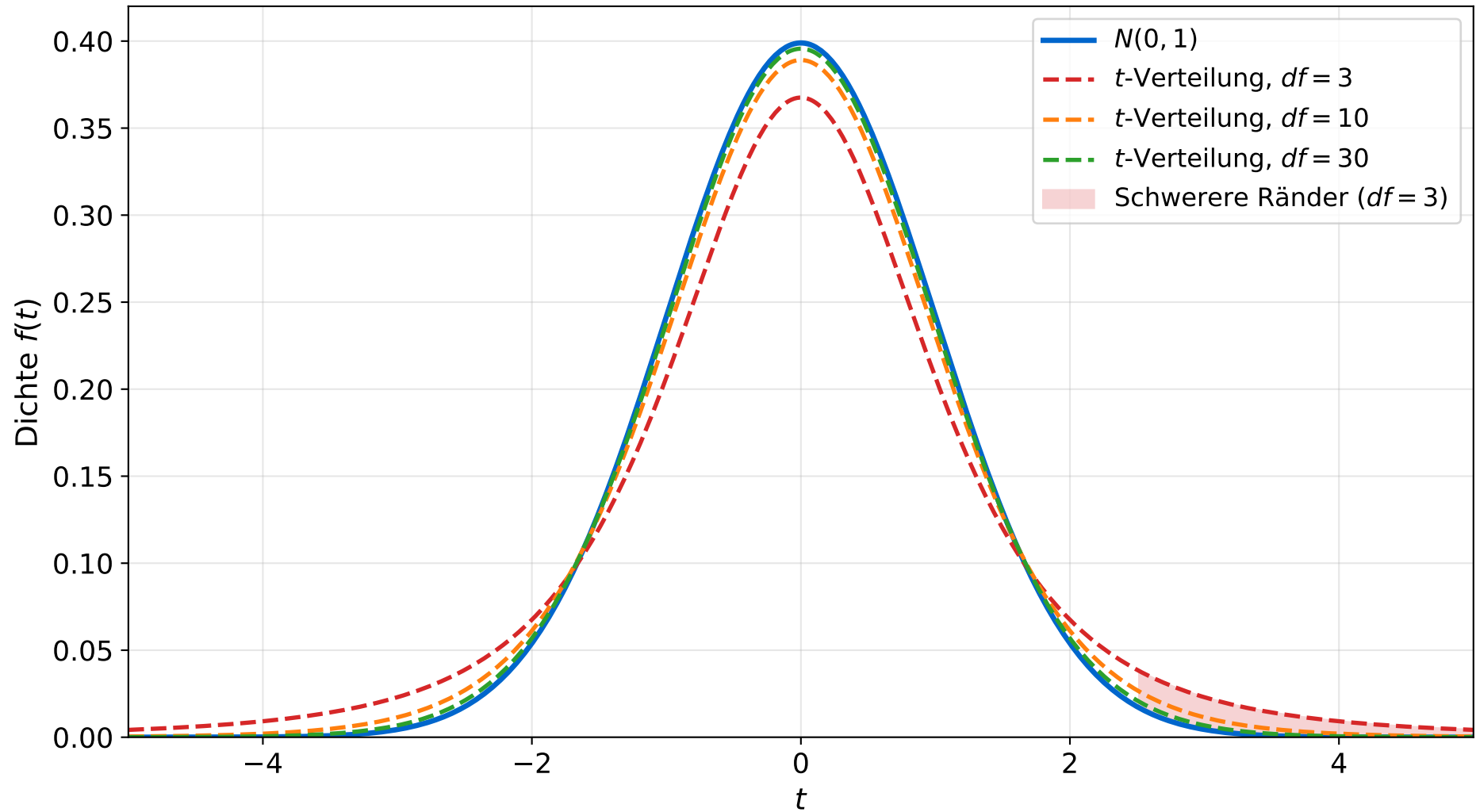
t -Verteilung vs. Standardnormalverteilung
