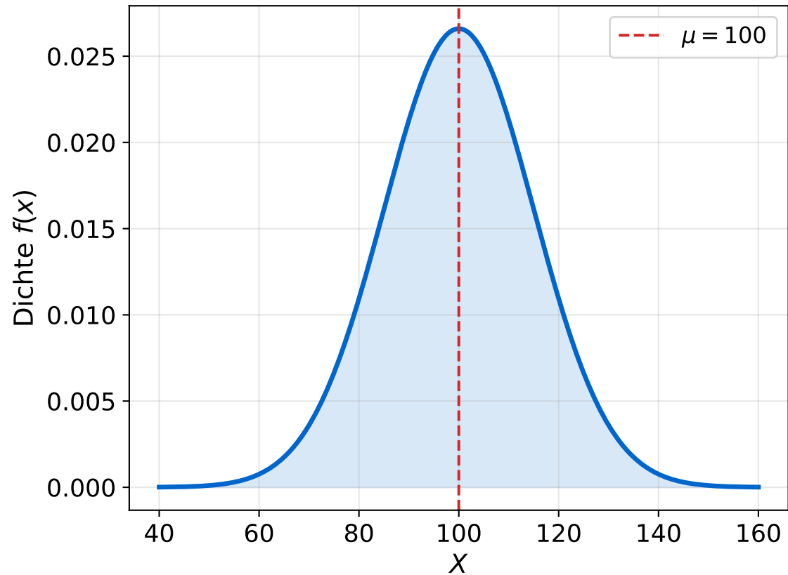
Grundgesamtheit: N(100, 15^2)
