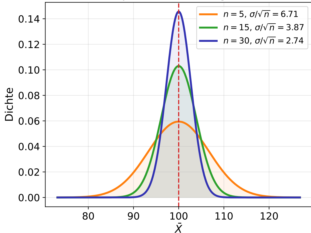
Stichprobenverteilung von \bar{X}
