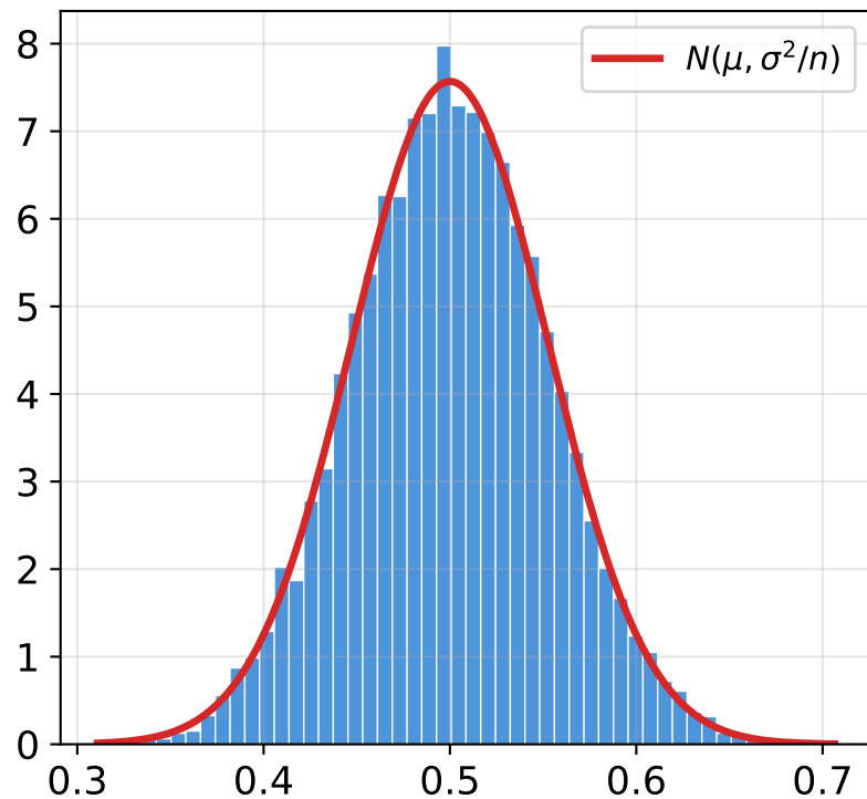
Gleichverteilung Uniform(0,1)
