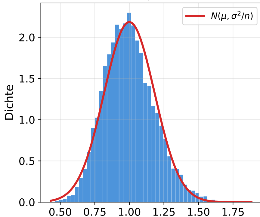
Exponentialverteilung Exp(1)
