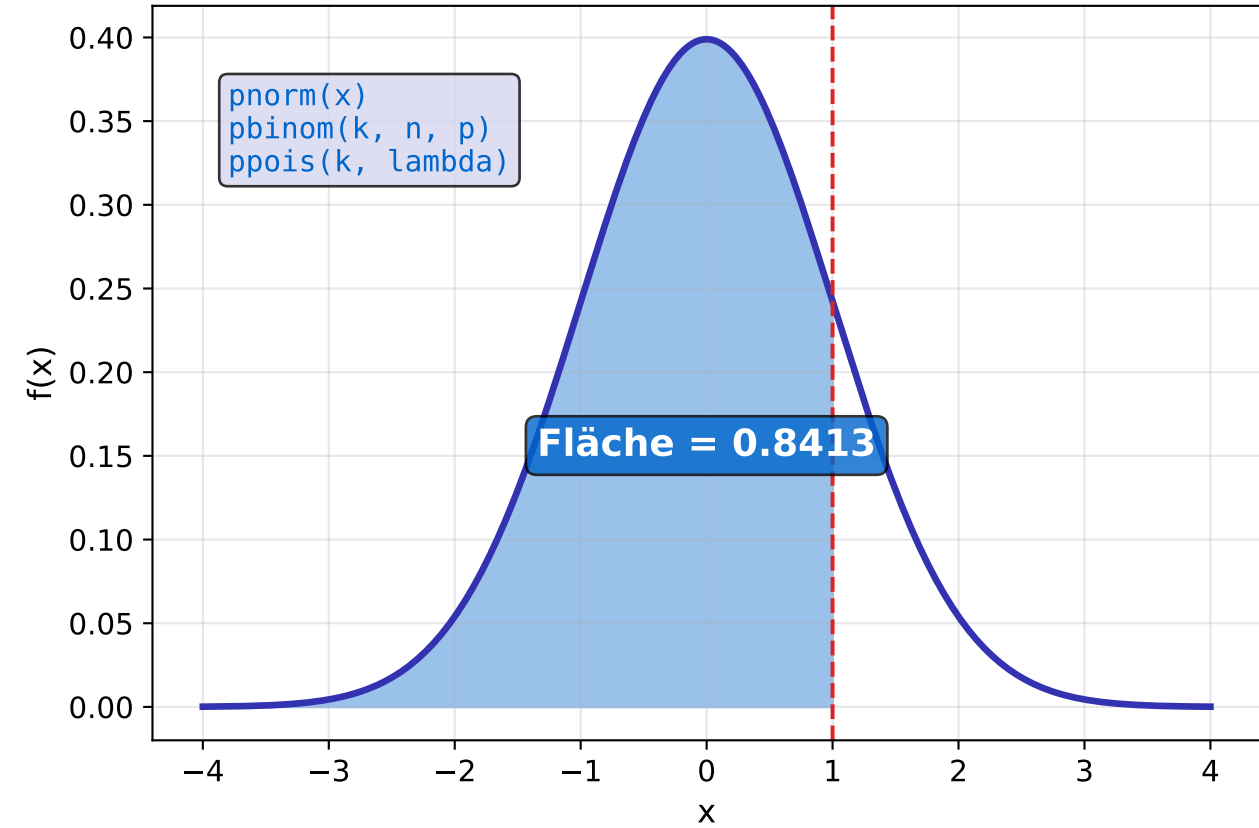
p-Funktion: P(X \leq x)
