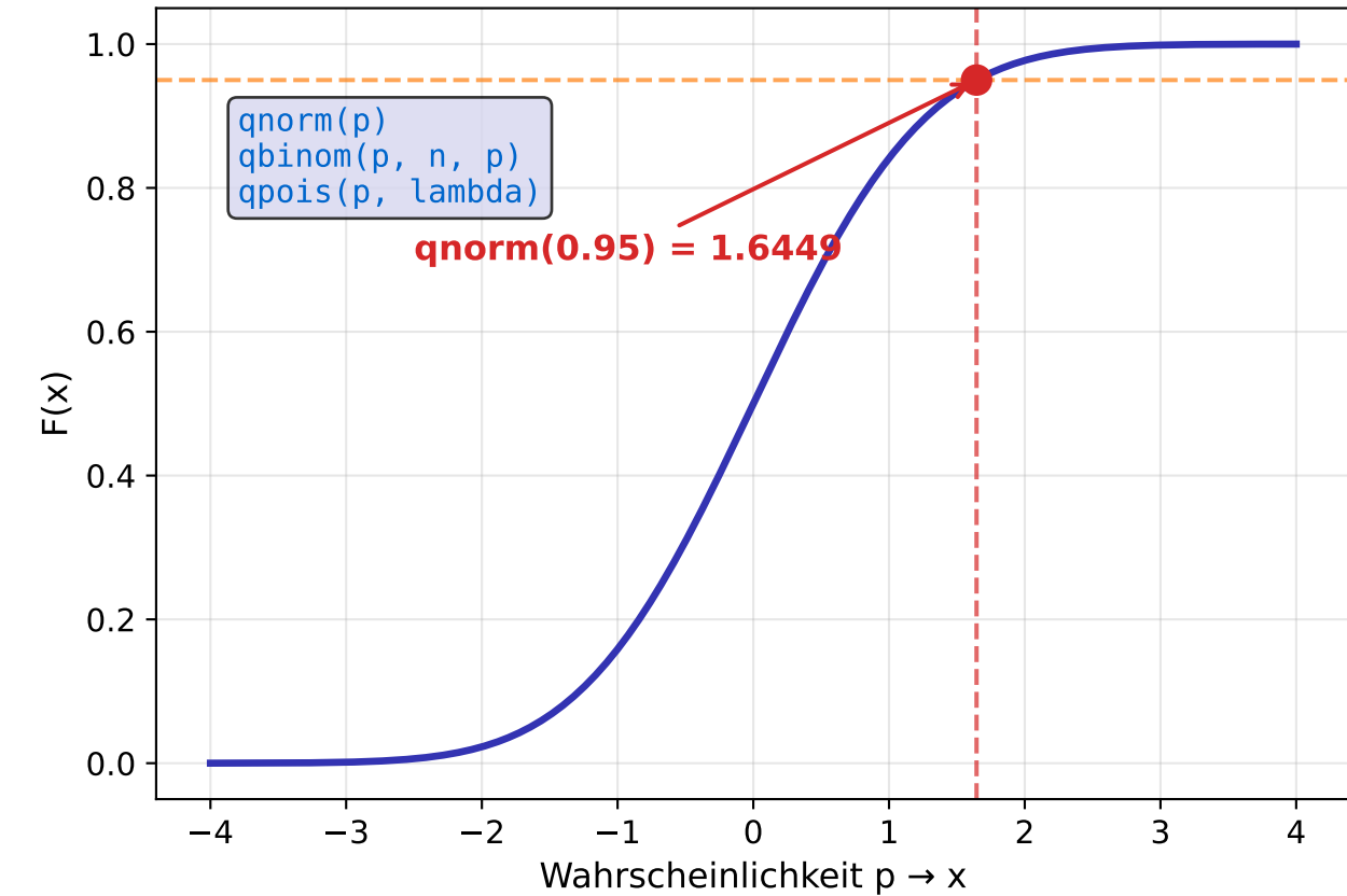
q-Funktion: Quantil (Umkehrung von p)
