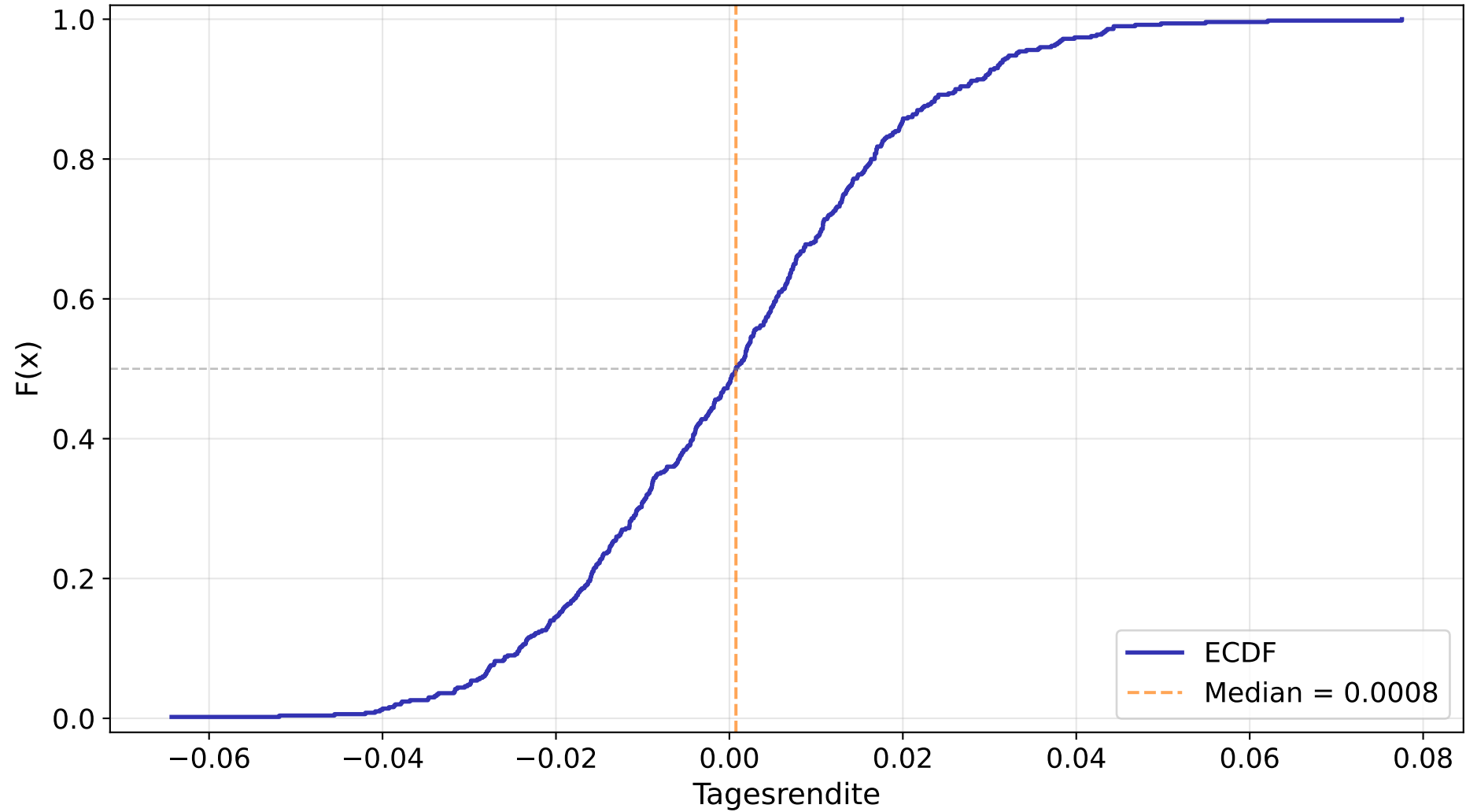
Empirische Verteilungsfunktion (ECDF) der Tagesrenditen
