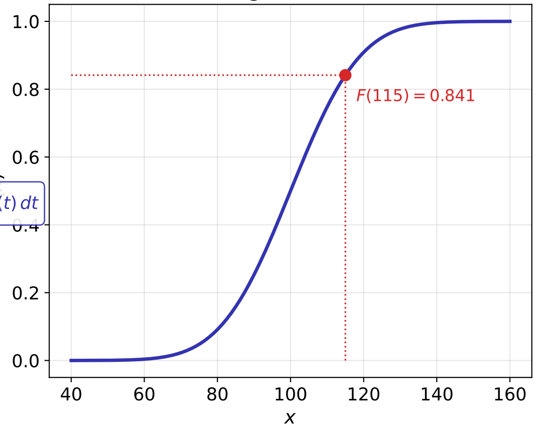
Verteilungsfunktion (CDF)
