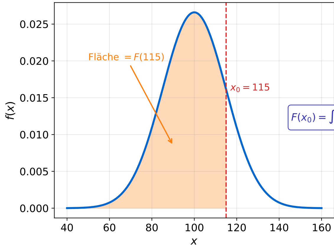
Dichtefunktion (PDF)
