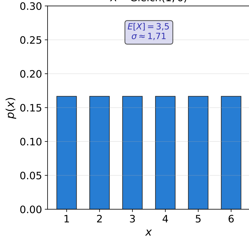
Gleichverteilung X \sim \text{Gleich}(1, 6)
