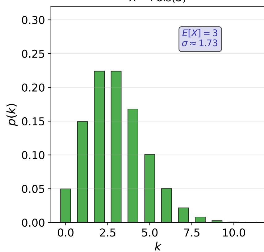
Poissonverteilung X \sim \text{Pois}(3)
