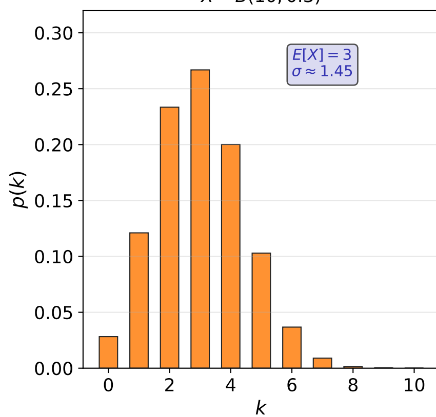
Binomialverteilung X \sim B(10, 0.3)
