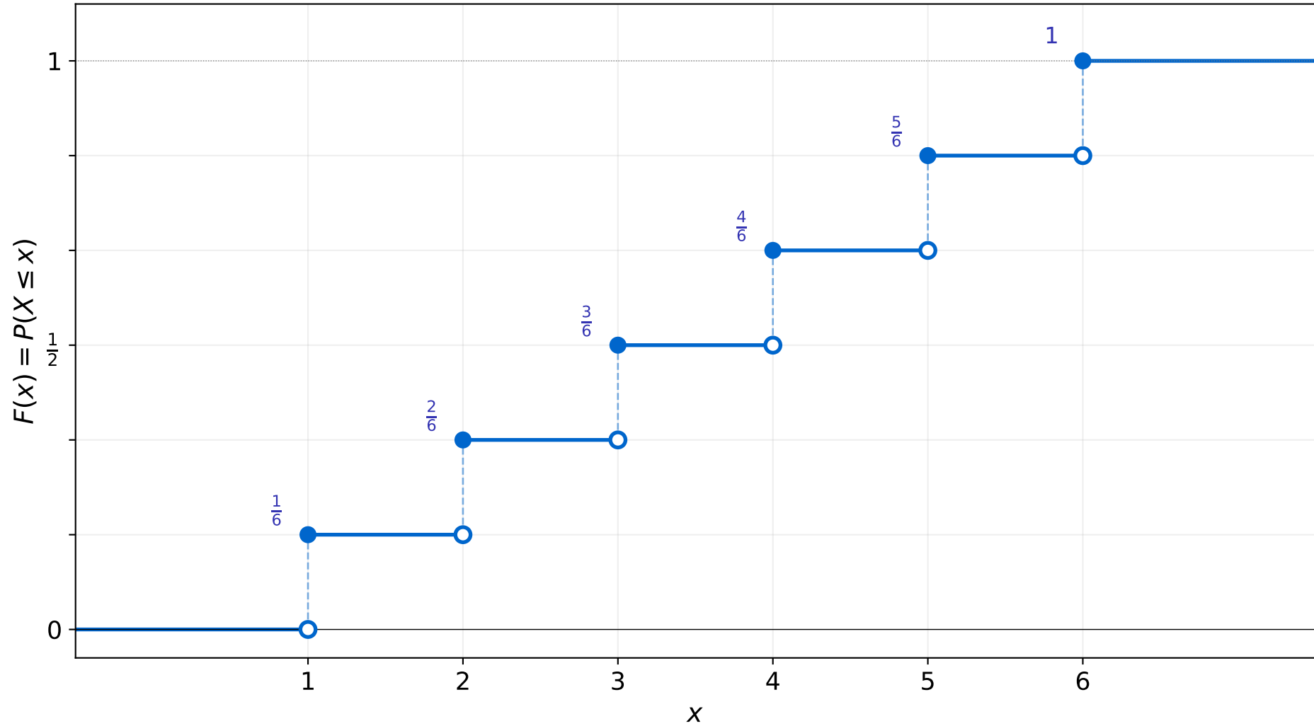
Verteilungsfunktion (CDF) eines fairen Würfels
