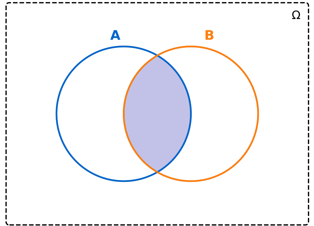
A \cap B (Schnitt)
