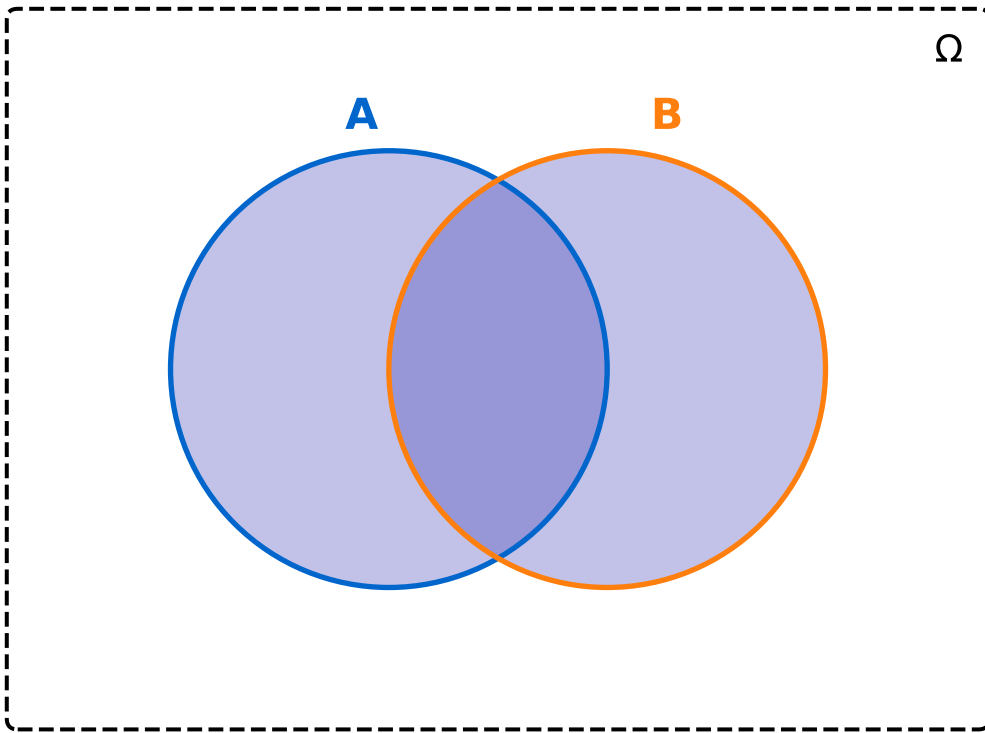
A \cup B (Vereinigung)
