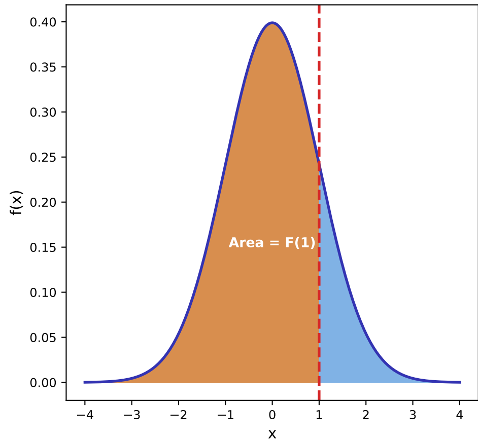
PDF: f(x)
