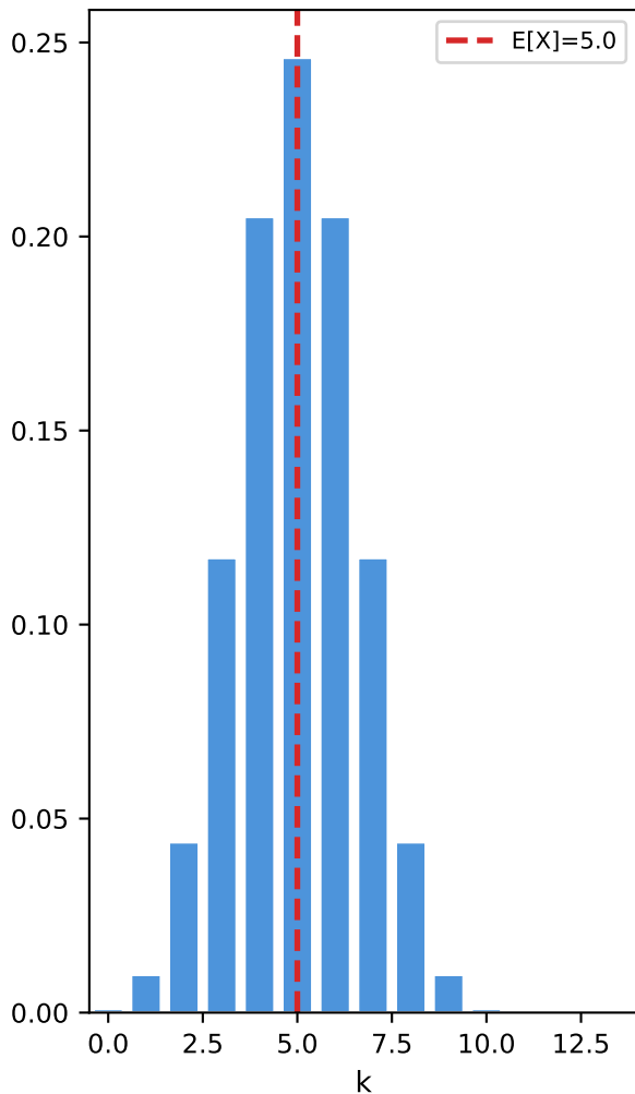
Binomial( n=10, p=0.5 )
