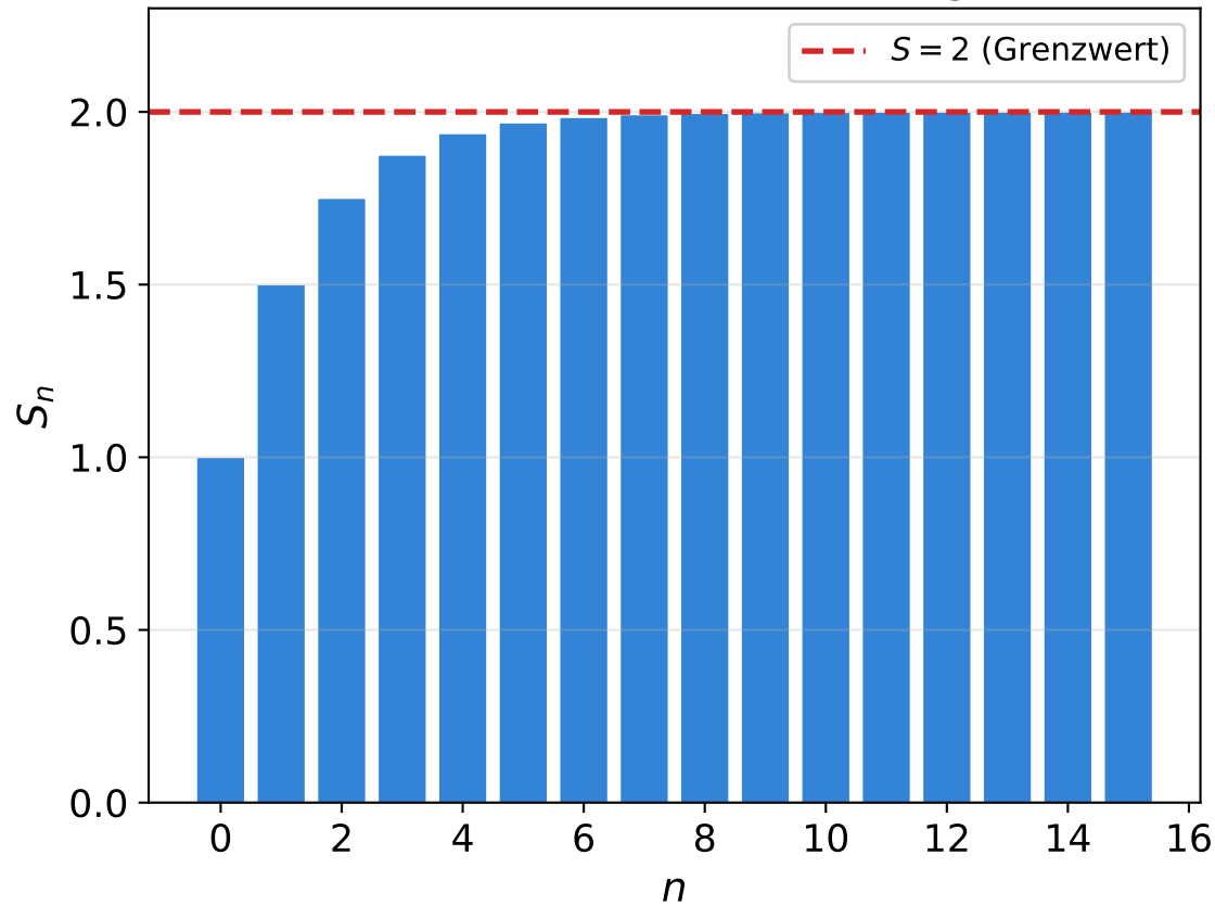
Geometrische Reihe (konvergent)
