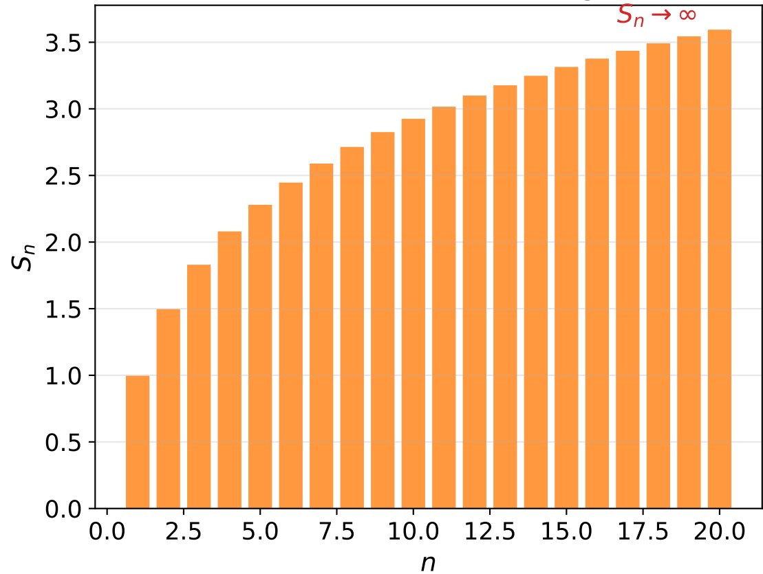
Harmonische Reihe (divergent)
