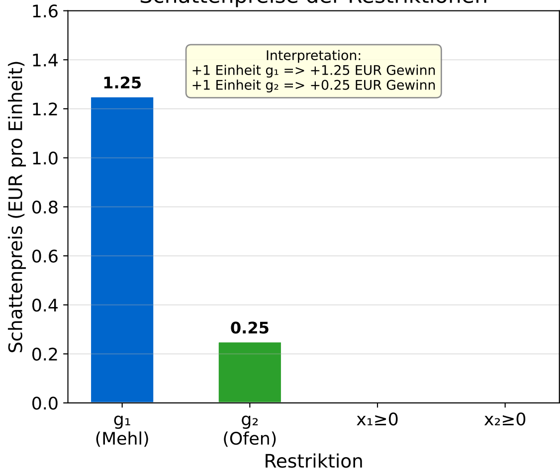
Schattenpreise der Restriktionen
