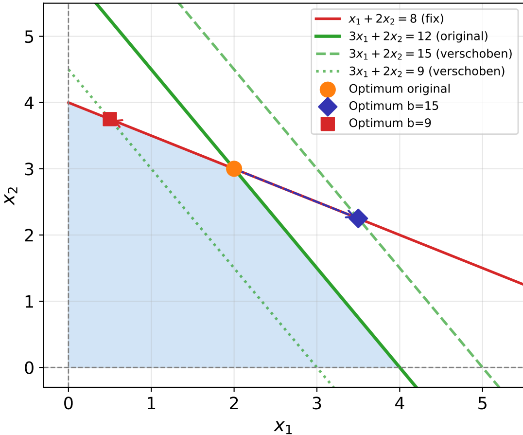
Verschiebung der Restriktion g_2
