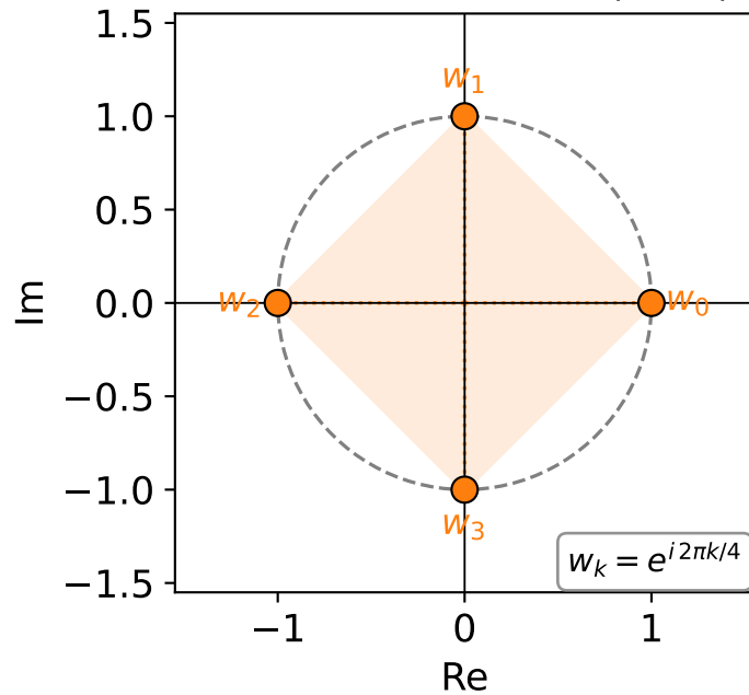
4-te Einheitswurzeln ( n = 4 )
