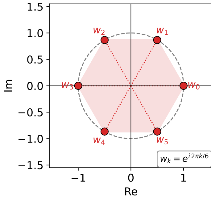
6-te Einheitswurzeln ( n = 6 )
