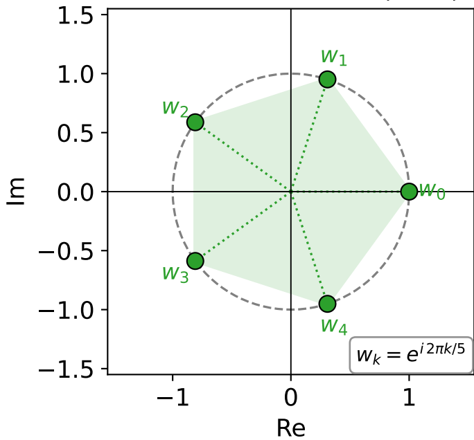
5-te Einheitswurzeln ( n = 5 )
