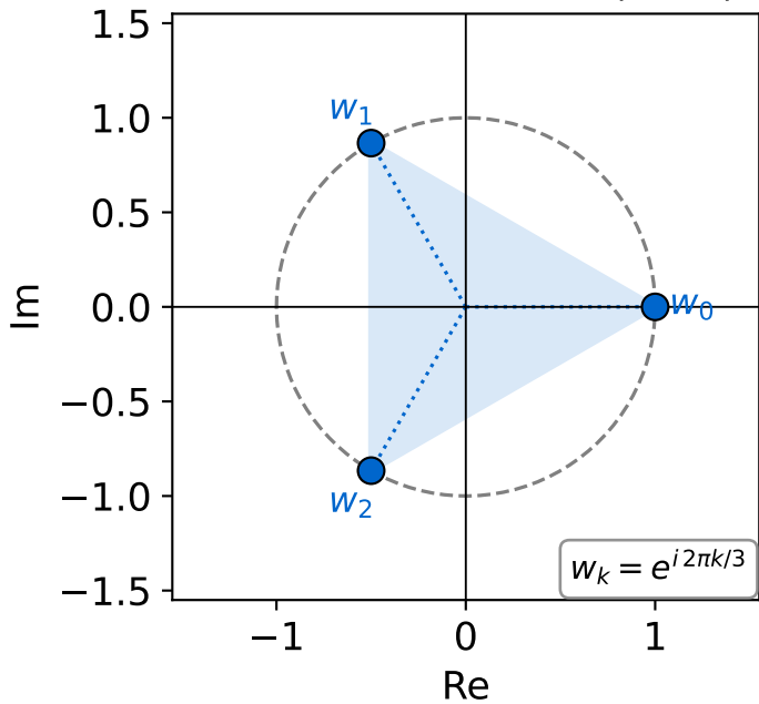
3-te Einheitswurzeln ( n = 3 )
